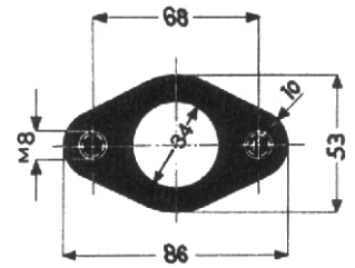
Flanschzeichnung
