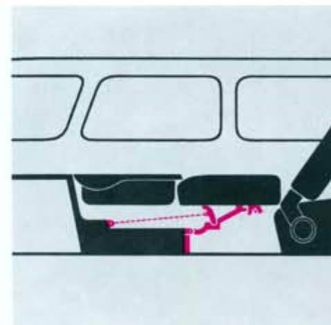
32. Stützscharnier , für Liegeeinrichtung im VW Variant. Schafft eine Liegefläche von 2,10 m Länge.
