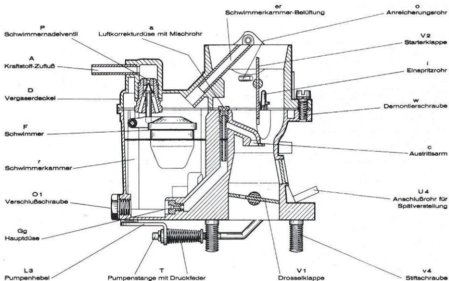
Bild 3: Solex-Fallstromvergaser 30, 31, 34 PICT-3 (schem. Schnitt)
