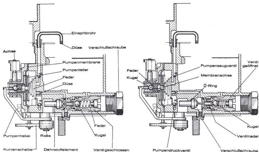
Bild 19: SOLEX-Fallstromvergaser 31 PICT-4 (schematischer Schnitt)
