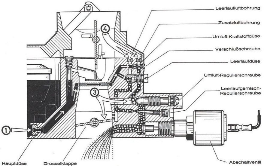
Bild 10: 34 PICT-3 Wirkungsweise des Leerlauf- und Umluftsystems
