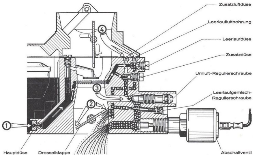
Bild 11: 30 und 31 PICT-3 Wirkungsweise beim Übergang
