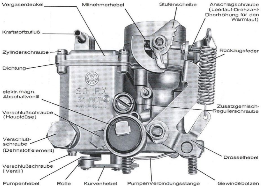
Bild 17: SOLEX-Fallstromvergaser 31 PICT-4
