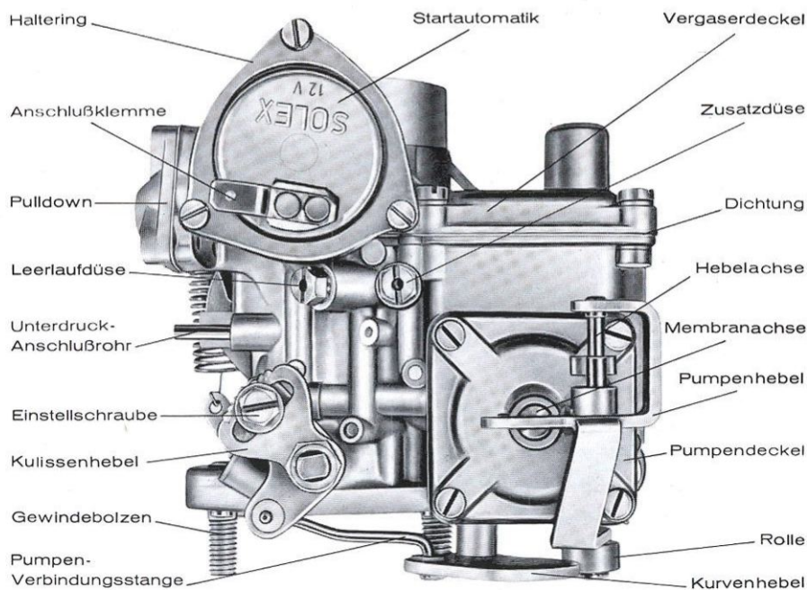
Bild 18: SOLEX-Fallstromvergaser 31 PICT-4
