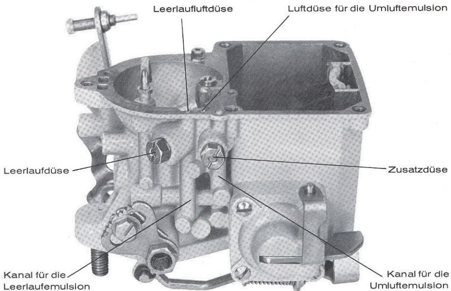
Bild 12: Vergasergehäuse 30 und 31 PICT-3 Kanalführung für das Leerlaufsystem links, für das Umluftsystem rechts.
