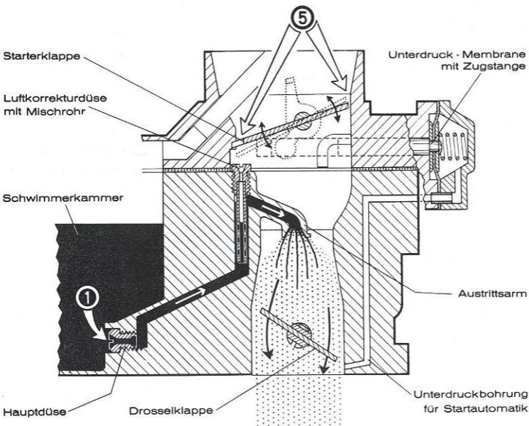
Bild 8: Wirkungsweise der Startautomatik beim Kaltstart
